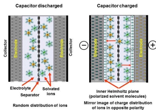
شکل ۱: ساختار مکانیزم EDLC در ابرخازن
