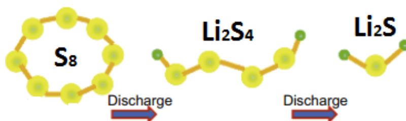
شکل ۸: واکنش سولفور با لیتیوم در فرآیند تخلیه (شارژ) باتری‌های لیتیوم-سولفور
