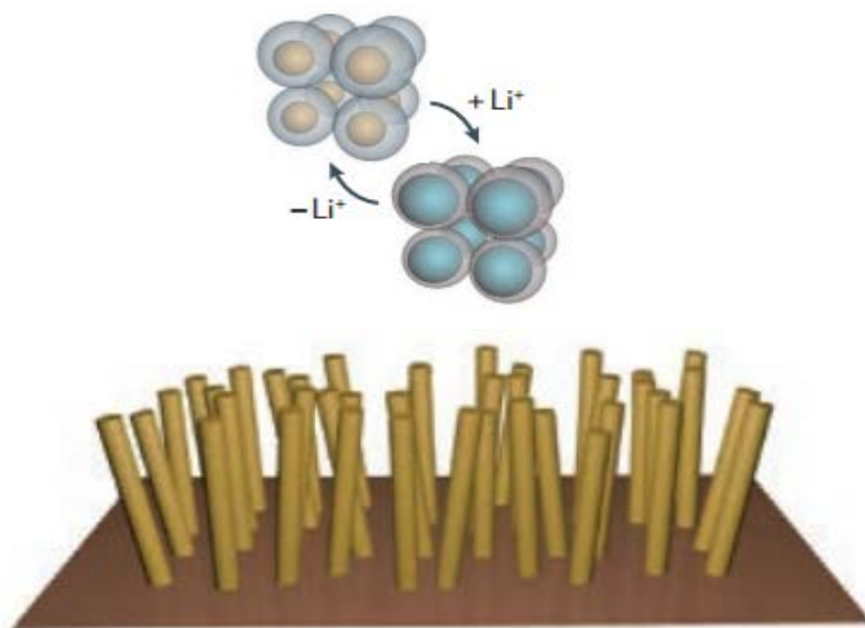
شکل ۵: بهبود آندهای سیلیکونی با استفاده از نانوسیم‌های سیلیکونی (سمت راست) و قرار دادن نانو ذرات سیلیکون درون محفظه‌های محافظ (سمت چپ)
